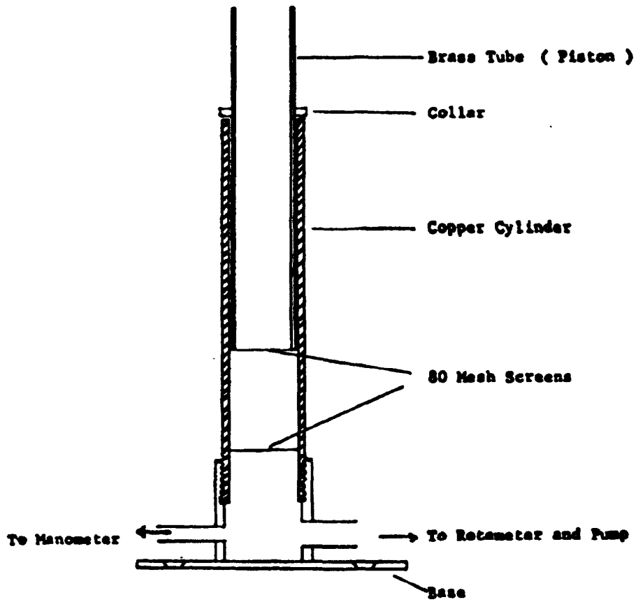
FIG. 1 GIPD APPARATUS
